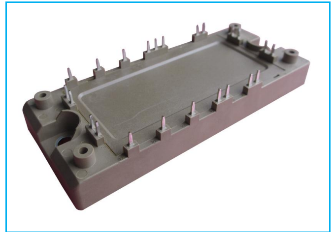
Rectifier+Brake+Inverter
